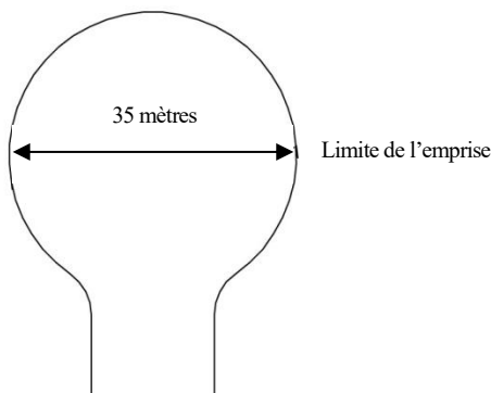
Illustration 10. Emprise d'un rond de virage.
